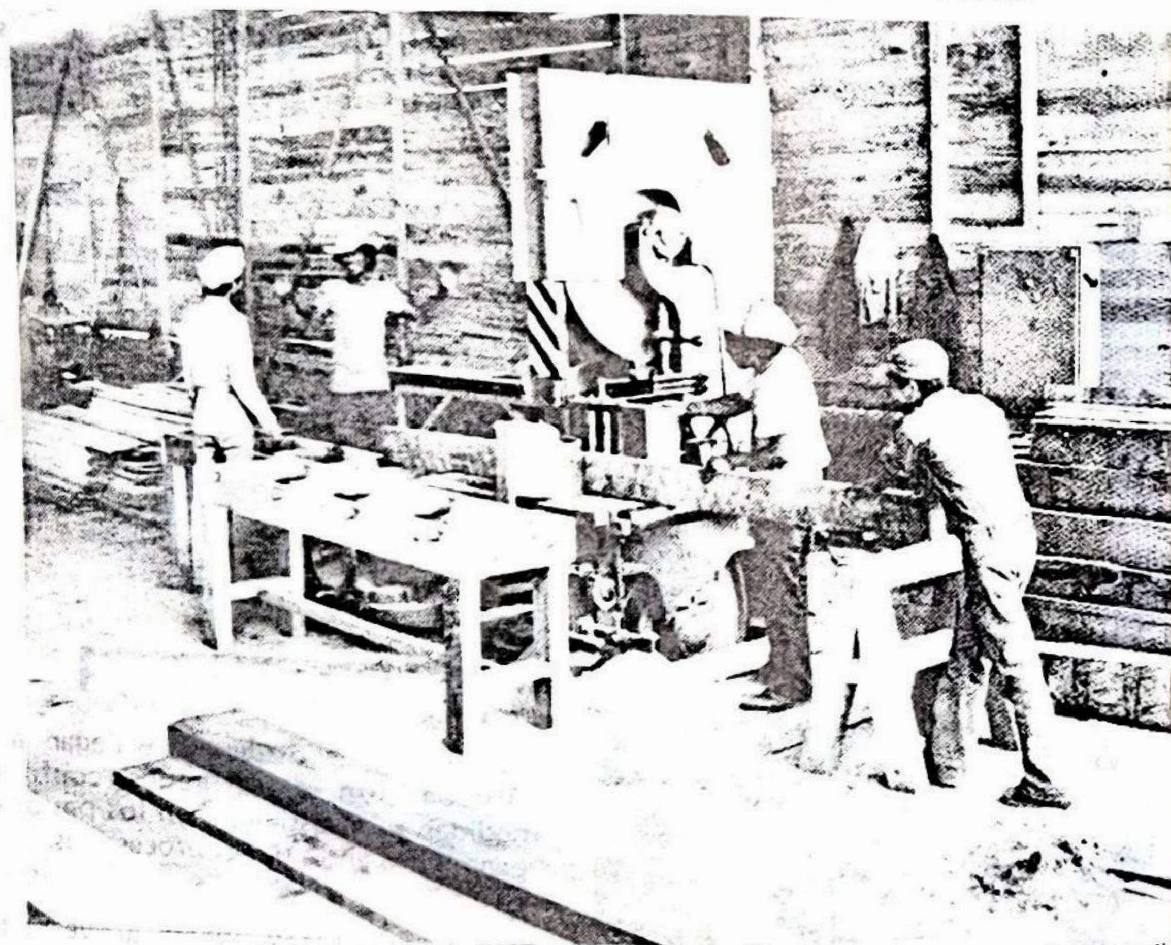
Los blocks de madera entran a la sierra de cinta de donde se obtienen duelas y tablones.
