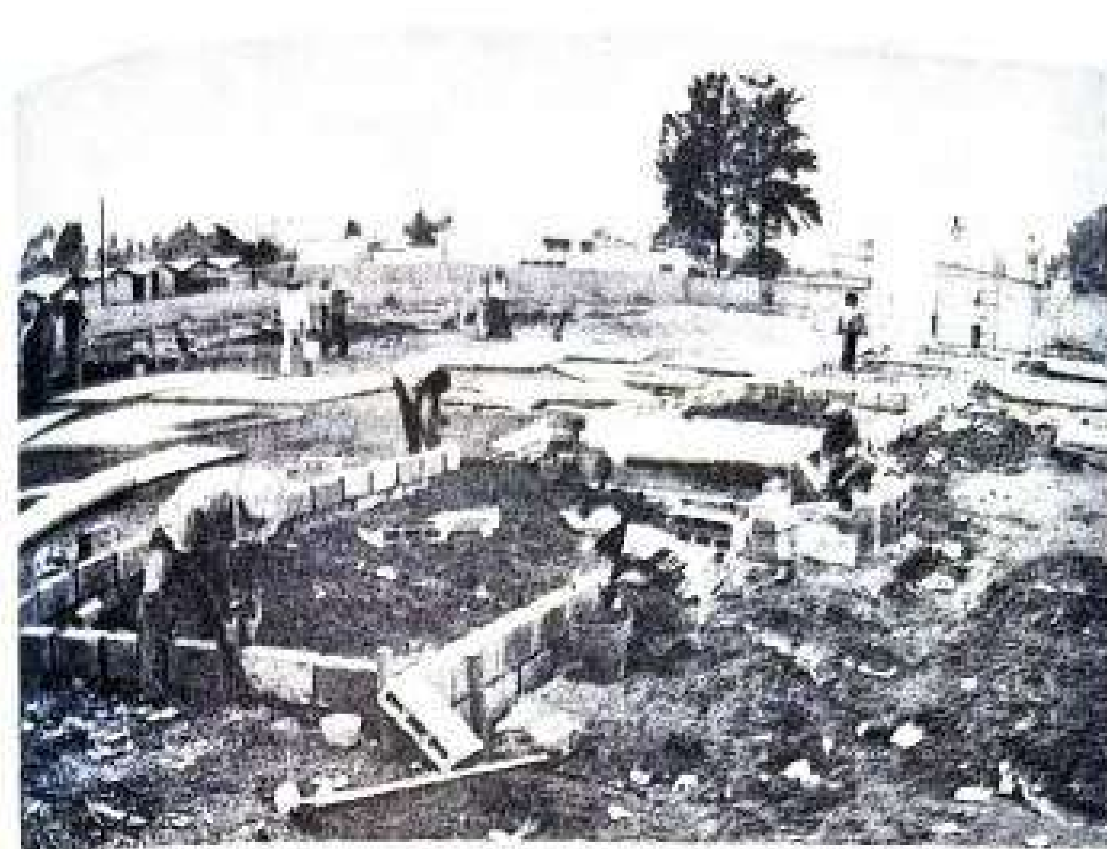
Proyecto IGSS - empleados del Instituto Guatemalteco de Seguridad Social (IGSS), construyen las bases en donde se levantarán las viviendas HODE, con asistencia social, técnica y financiera de Hode.
