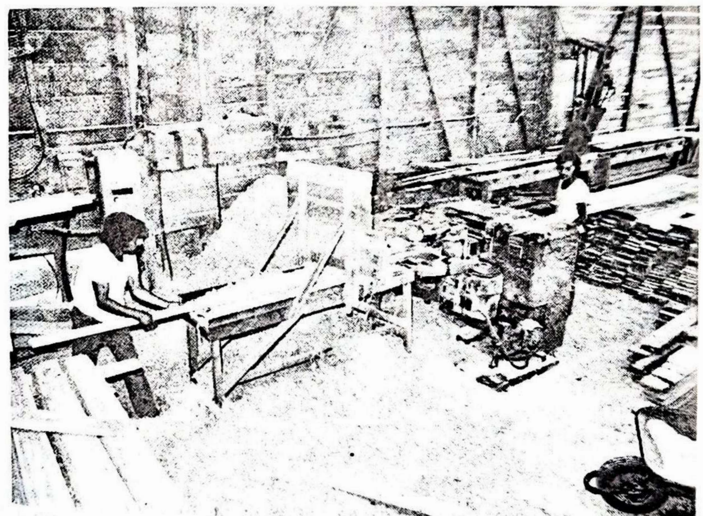
Las duelas de madera, a su vez, son convertidas en machihembre tipo bota-agua, en esta máquina.
