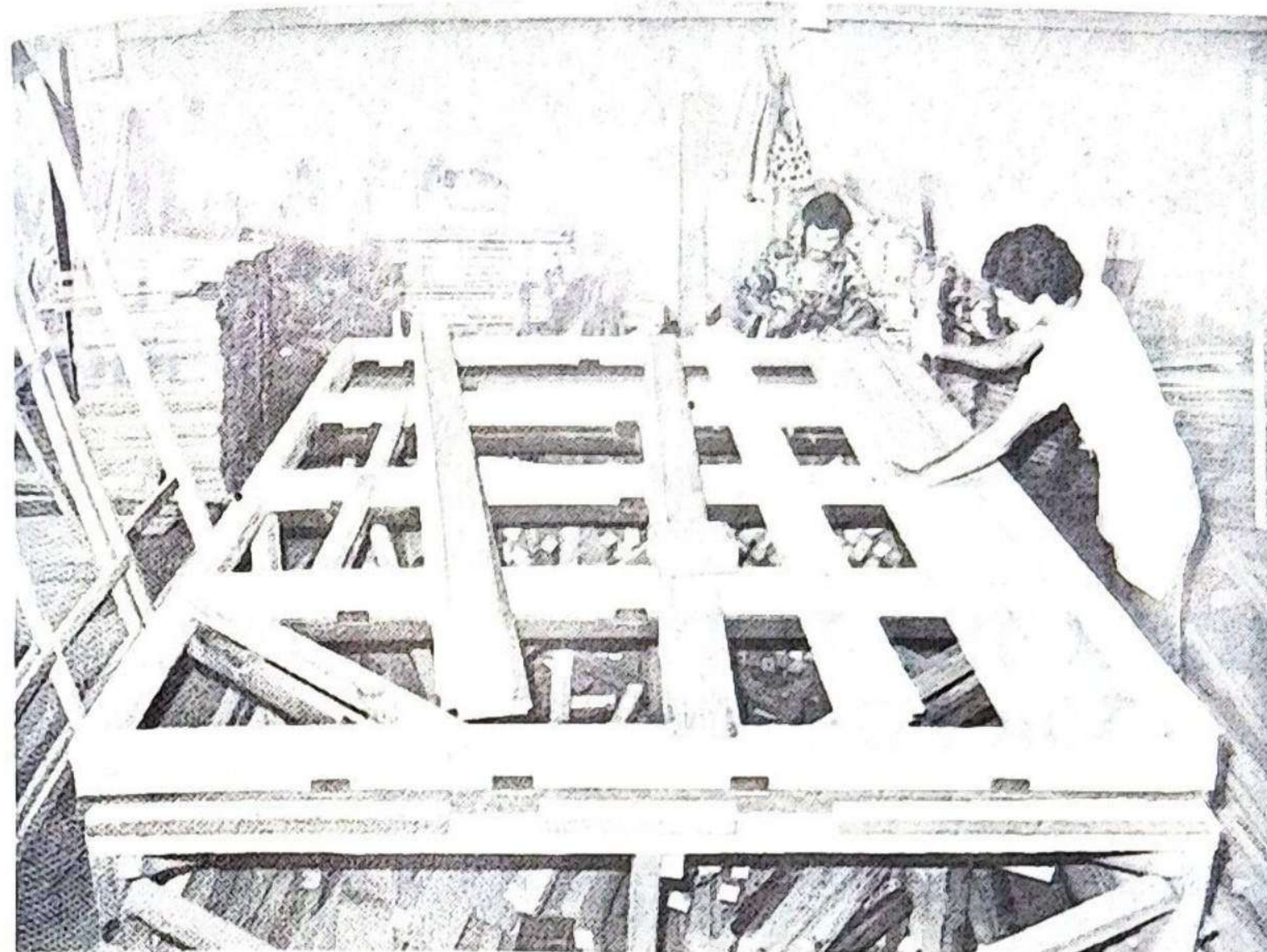
Con las duelas de machihembre precortadas se forran las armazones de los paneles.
